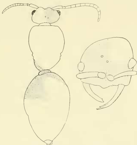
Fig. 1. Dasyutilla euchroa Ckll., gynandromorph.
